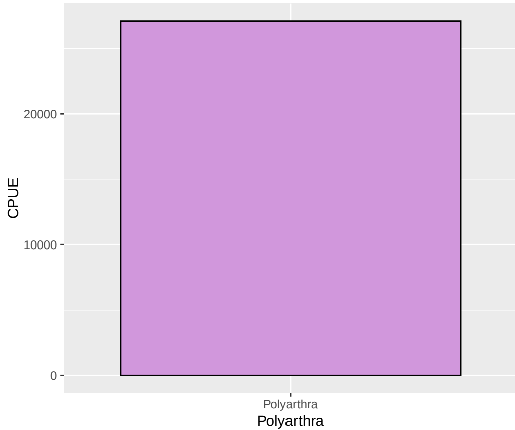
CPUE of Polyarthra
